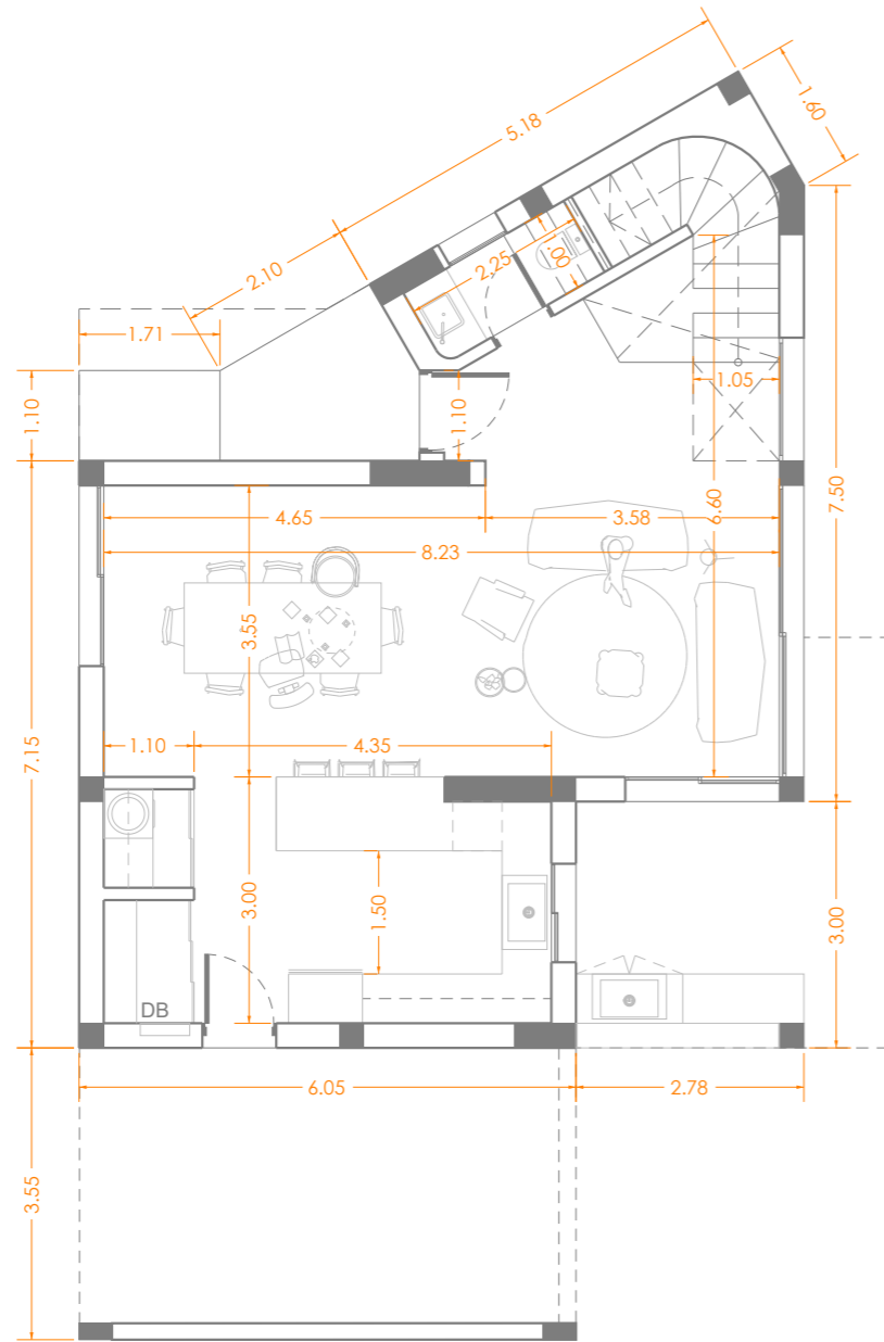
ΚΑΤΟΨΗ ΙΣΟΓΕΙΟ
