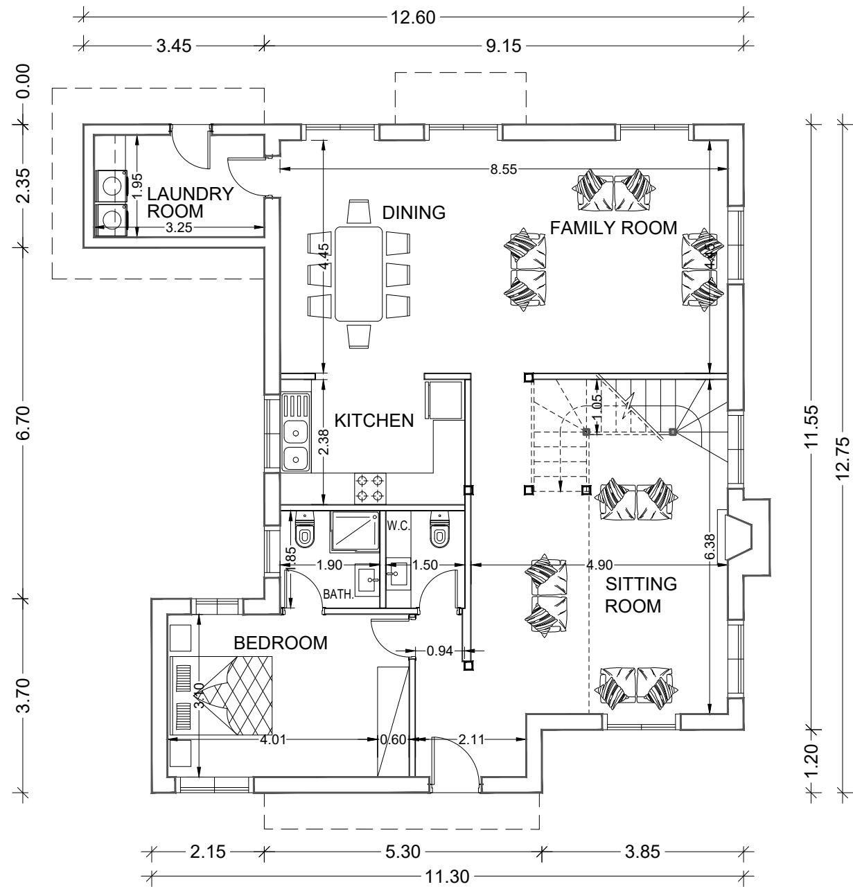
ΚΑΤΟΨΗ ΙΣΟΓΕΙΟΥ
