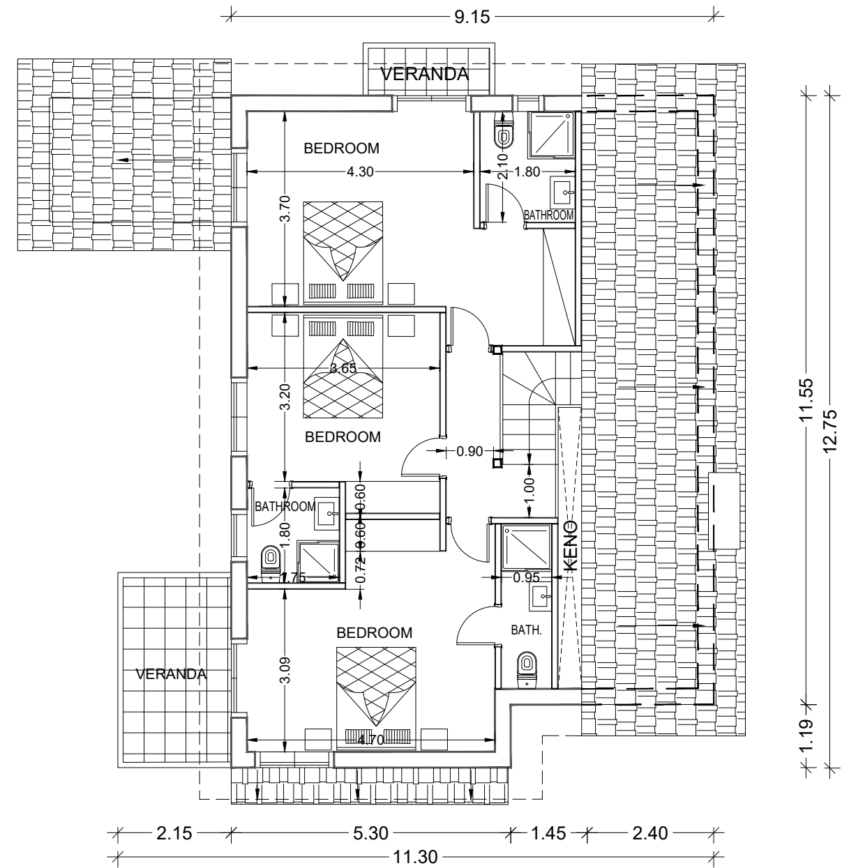
ΚΑΤΟΨΗ ΟΡΟΦΟΥ
