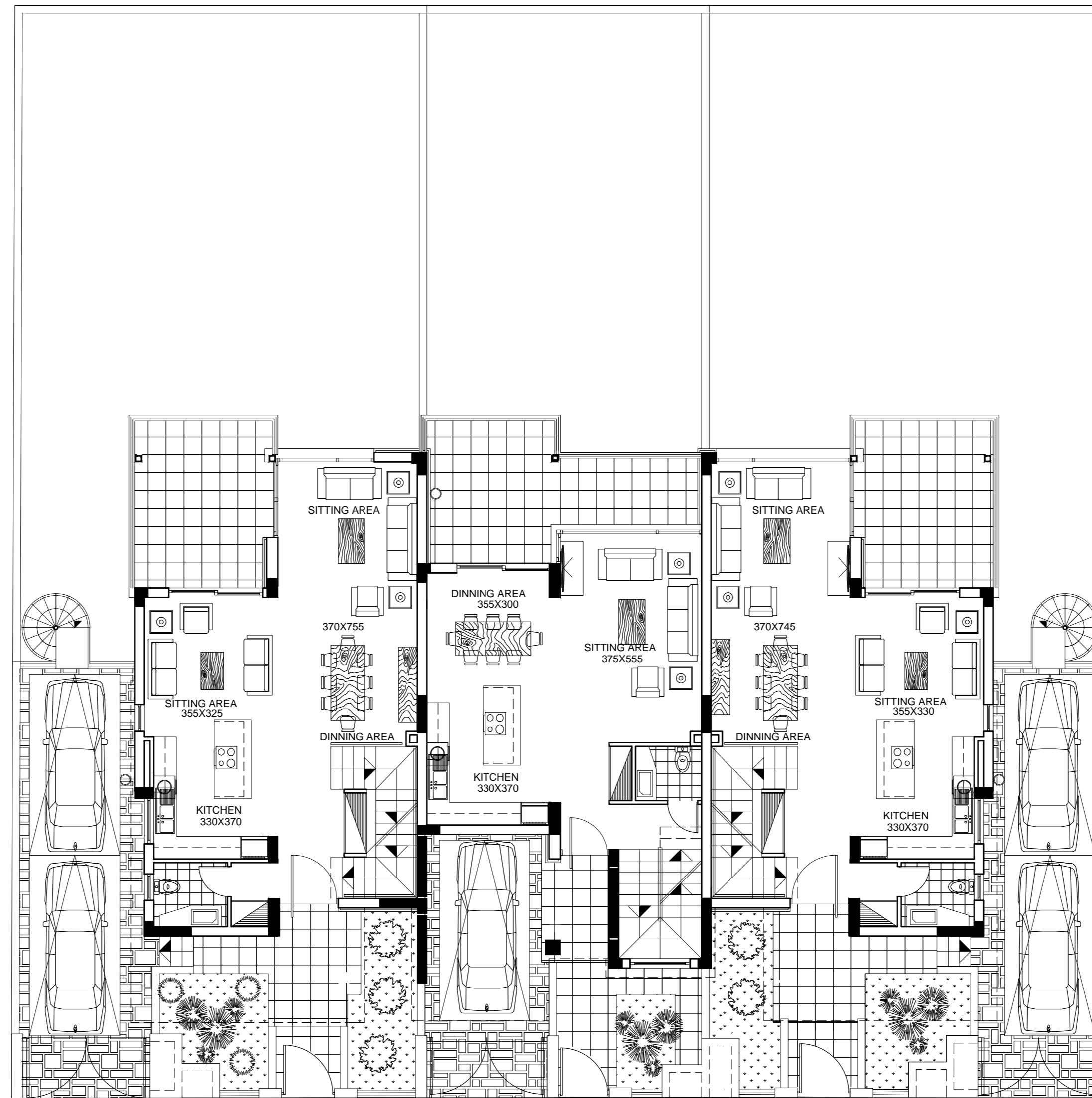
maisonette 1
