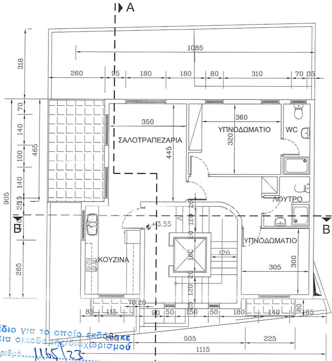
ΚΑΤΟΨΗ 1ου ΟΡΟΦΟΥ
