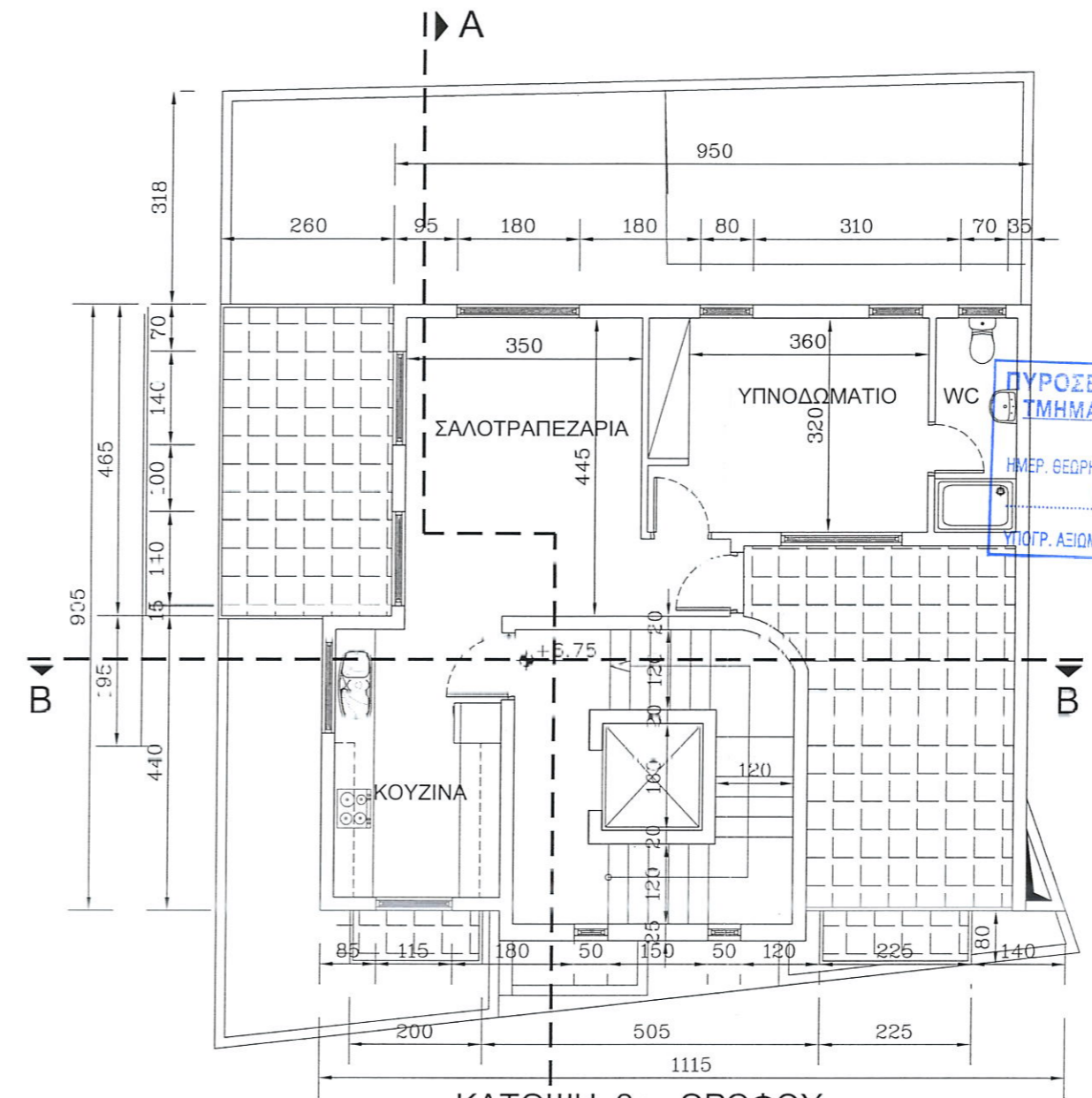
ΚΑΤΟΨΗ 2ου ΟΡΟΦΟΥ
