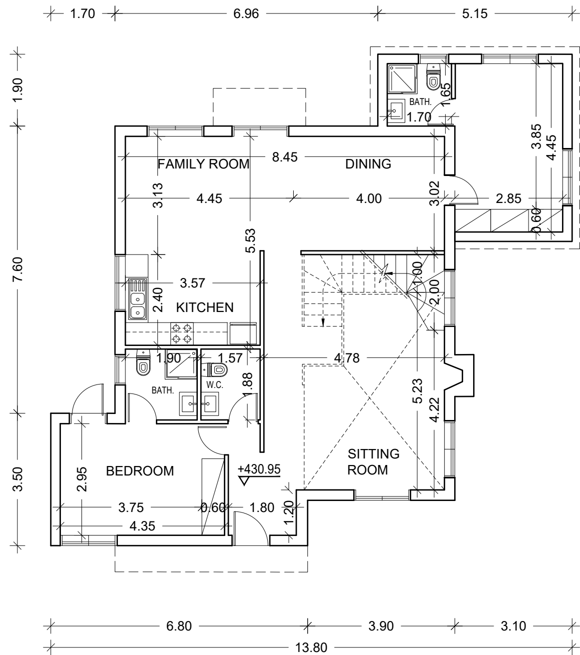
ΚΑΤΟΨΗ ΙΣΟΓΕΙΟΥ
